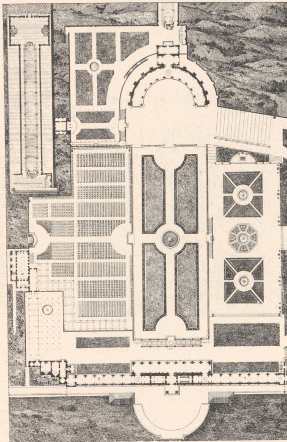
Abb. 276 Villa Albani, Rom, Grundriß des Gartens zwischen Kasino und Kaffeehaus ohne den seit- lichen Park
