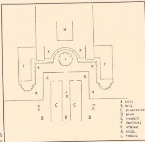
Abb. 72 Römische Villa, Grundriß zu Abb. 71
