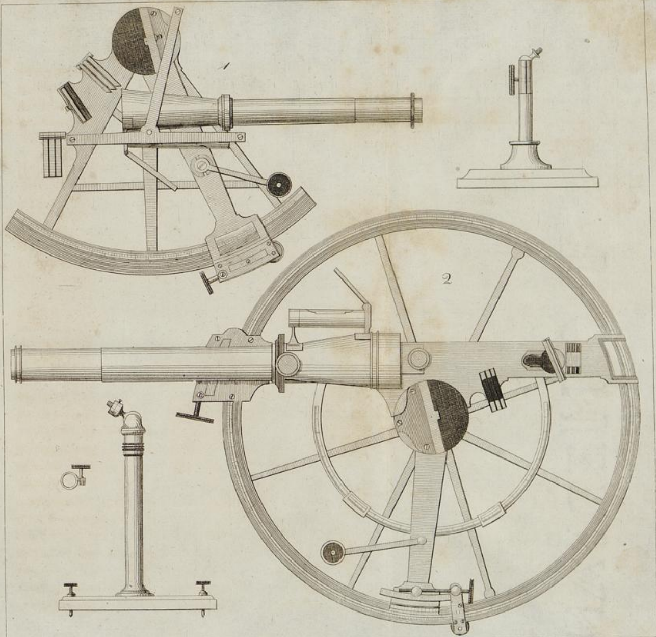
1. Hadleys Spiegelsextant. 2. Mayers Spiegelkreis.
