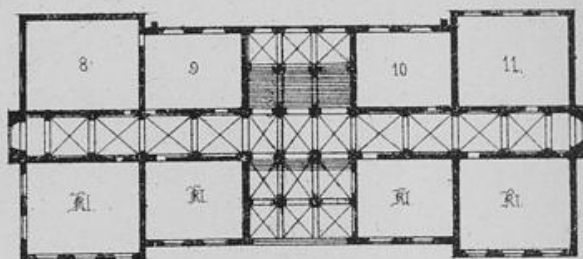
Erstes Geschoss
