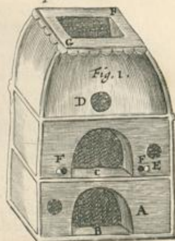
Furnus apertus probatorius
