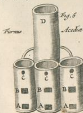
Pyxis seu tegula cæmentatoria
