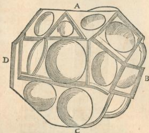
Figura I. Dodecaedri.
