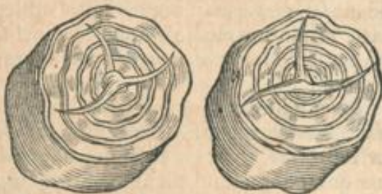
Fig. II.
