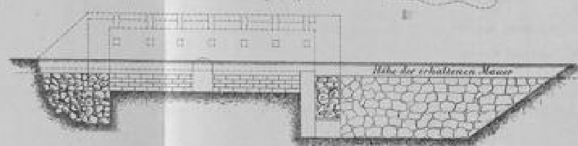
Fig. V. Schnitt nach e. f. (Fig. 13)
