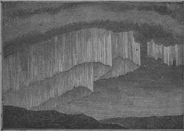
Mantelförmiges Nordlicht, im Winter 1838–1839 zu Bossekop von Schiffalleutnant Lottin beobachtet.
