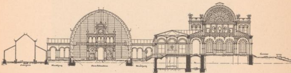
Vorderschnitt
