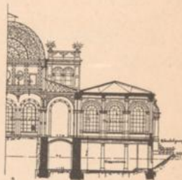
Schnitt C-D
