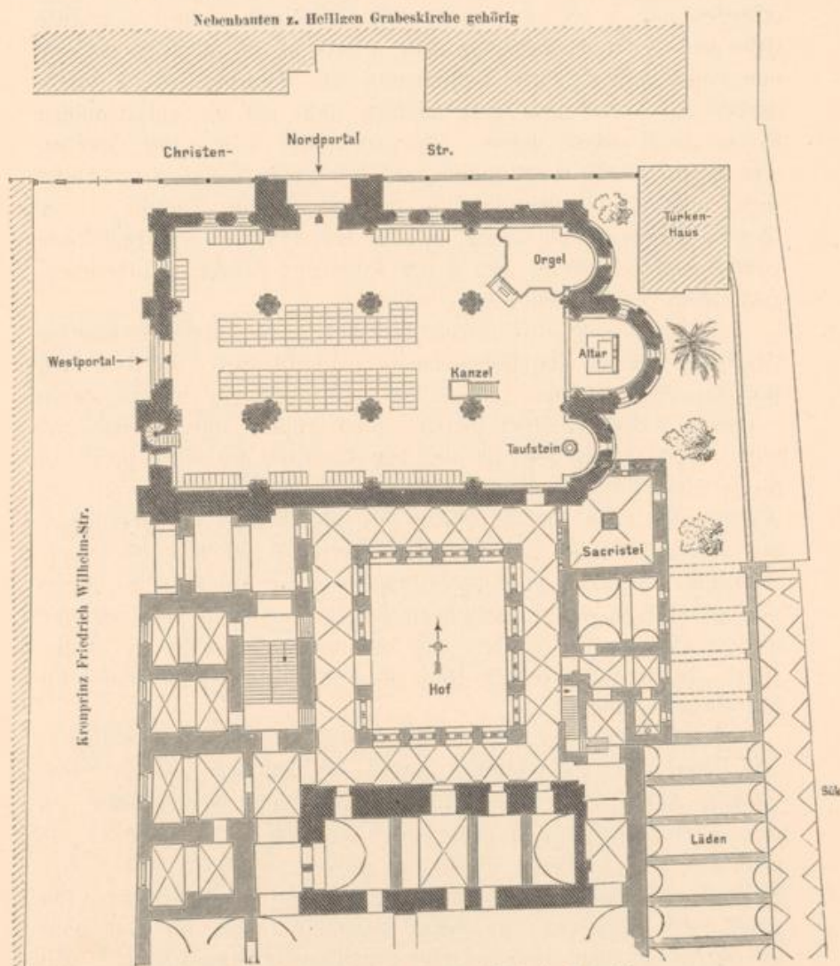
Grundriß der evangelischen Erlöserkirche in Jerusalem.
