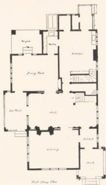
ARCH. WILLIAM E. STONE • GRUNDRISS ZUM LANDHAUS IN PRINCETON (VGL. SEITE 190)
