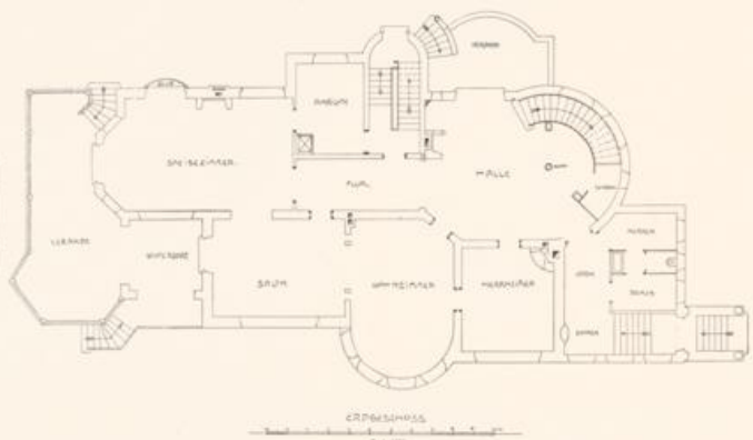
GRUNDRIßZ DES HAUSES ENGLÄNDER (VGL. SEITE 33 UND 35)
