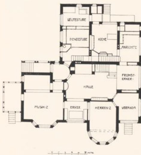
ARCH. DR. ING. HERM. MUTHESIUS-BERLIN • HAUS VON SCHUCKMANN IN ZEHLENDORF-WEST: LAGEPLAN, GARTENANLAGE UND GRUNDRISS (VOL. SEITE 29) (BAUKOSTEN, OHNE GARTEN 65000 Mk.)
