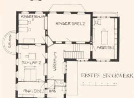
ARCH. DR. ING. HERMANN MUTHESIUS • HAUS SEEFELD IN ZEHLENDORF: LAGEPLAN, GARTENANLAGE UND GRUNDRISS (VOL. SEITE 31. BAUKOSTEN MIT GARTEN UND EINFRIEDIGUNG 45000 Mk.)
