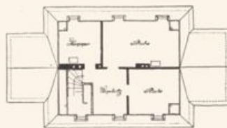
GRUNDRIß ZUM GÄRTNERHAUS DR. WENDELSTADTS IN GODESBERG (VGL. SEITE 57)
