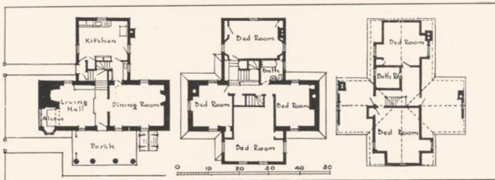
GRUNDRISS EINES KLEINEN AMERIKANISCHEN LANDHÄUSCHENS
