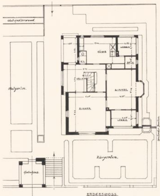
LAGEPLAN UND GRUNDRIß DES HAUSES E. BEUTINGER IN HEILBRONN (VGL. SEITE 62; BAUKOSTEN OHNE GARTENANLAGE UND UMZÄUNUNG 20 000 Mk.)
