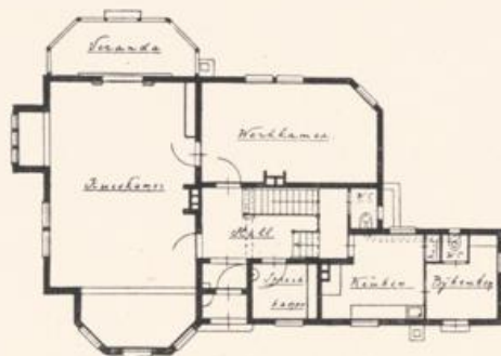
H. B. BERLAGE • GRUNDRISZ DES LANDHAUSES IN LAREN (VGL. SEITE 129)
