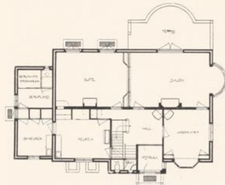
ARCH. JOS. TH. J. CUYPERS UND JAN STUYT-AMSTERDAM GRUNDRISSE ZU DEN LANDHÄUSERN IN BLOEMEN- DAAL UND AERDENHOUT (VGL. SEITE 133) •••••
