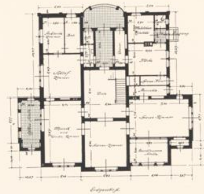
ARCH. REG.-BAUMEISTER PAUL MEBES-BERLIN GRUNDRISS ZUM HERRENHAUS „ST. HUBERTUS“ (VGL. SEITE 17)
