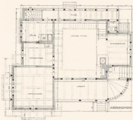
ARCH. DUŠAN JURKOVIČ-SEBROWITZ b. BRÜNN GRUNDRISS VOM ERDGESCHOSZ DES LANDHAUSES IN RESEK (VGL. SEITE 125)
