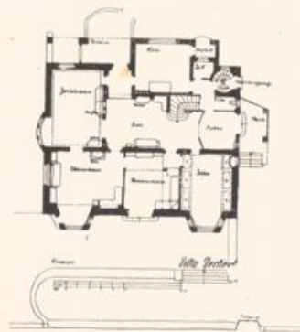
GRUNDRISZ ZUR VILLA DECKERT (VOL. SEITE 47)
