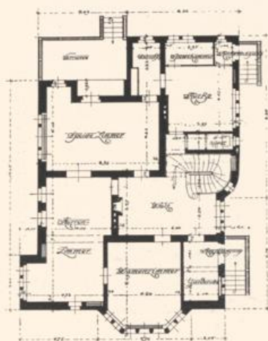
BAURAT DR. ING. ALFRED MESSEL- BERLIN ***** HAUS DR. BACK IN DARMSTADT: STRASZENSEITE UND GRUNDRISSSE VON ERD- UND OBER- GESCHOSZ *****
