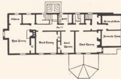
ARCH. WILSON EYRE • GRUNDRISS ZUM HAUS IN GREAT NECK (VGL. SEITE 180) • •
