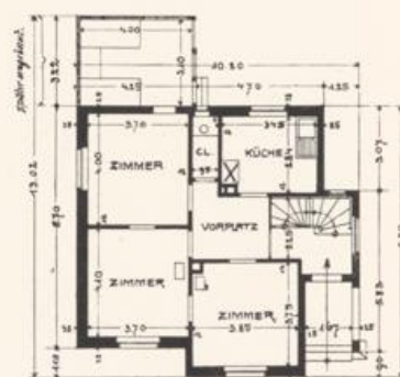
GRUNDRIß DES HAUSES GMELIN (BAUKOSTEN 10 000 Mk.)
