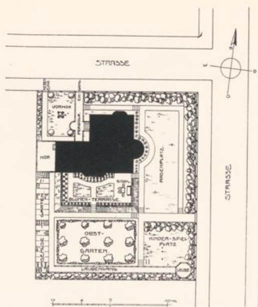
ARCH. DR. ING. HERMANN MUTHESIUS • HAUS SEEFELD IN ZEHLENDORF: LAGEPLAN, GARTENANLAGE UND GRUNDRISS (VOL. SEITE 31. BAUKOSTEN MIT GARTEN UND EINFRIEDIGUNG 45000 Mk.)
