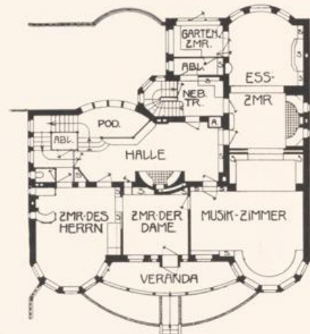
HAUS BERNHARD, GRUNEWALD BEI BERLIN, STRASZEN- SEITE UND GRUNDRISSSE (LAGEPLAN SIEHE SEITE 26) (BAUKOSTEN, EINSCHLIESZLICH GARTENANLAGE UND EINFRIEDIGUNG, 150 000 Mk.)
