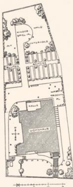
BAUINSPEKTOR ERICH BLUNCK • LAGEPLAN UND GRUNDRISS DES LANDHAUSES E. BLUNCK IN NIKOLASSEE (VGL. SEITE 27; BAUKOSTEN, OHNE GARTENANLAGE, 50000 Mk.)
