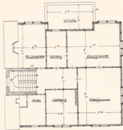
ARCH. REG.-BAUMEISTER KARL CAESAR-BERLIN • GRUNDRISS ZUM HAUS RUPRECHT (VGL. SEITE 15)
