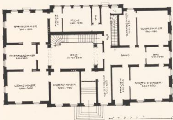
● GRUNDRIß ZUM LANDHAUS SCHUSTER IN MARKNEUKIRCHEN (BAUKOSTEN, EINSCHLIEßLICH GARTENANLAGE, 90.000 Mk.)
