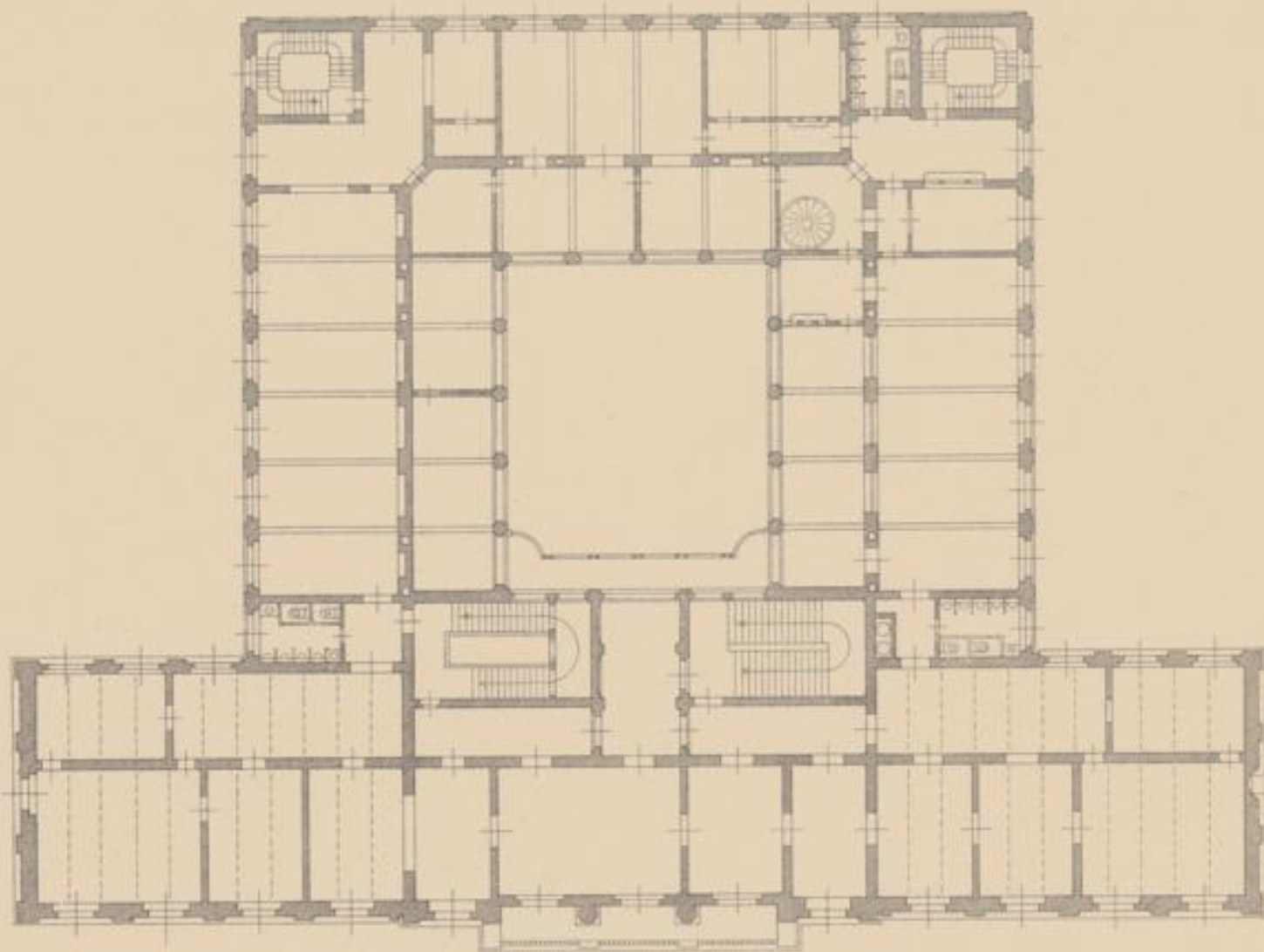
Erdgeschoss
