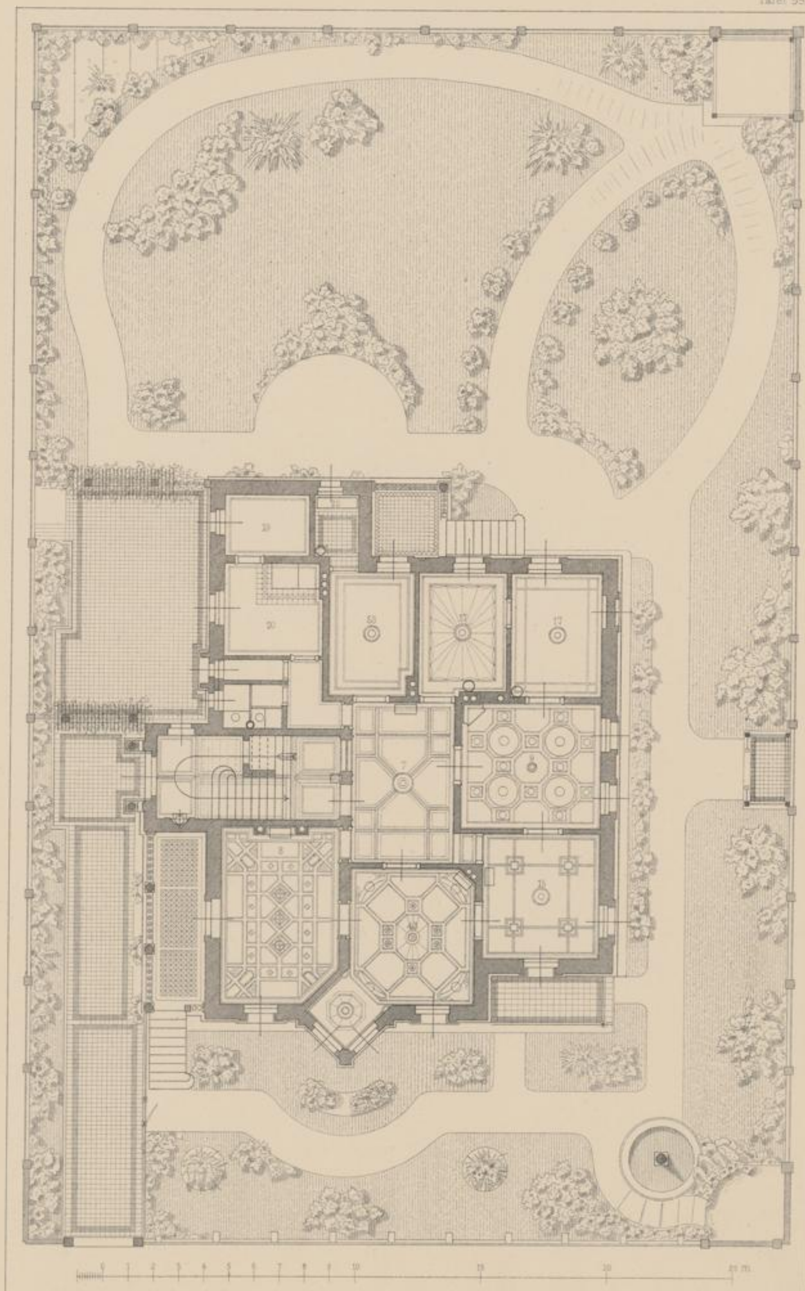
DRESDEN Villa Haensel - Eliasstrasse Plan - Grundriss - Groundplan
