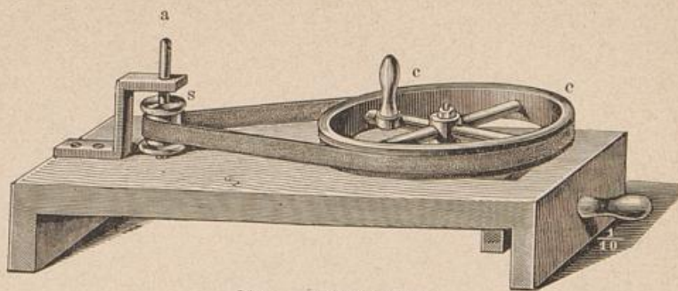
Fig. 1. Centrifugalmaschine.
