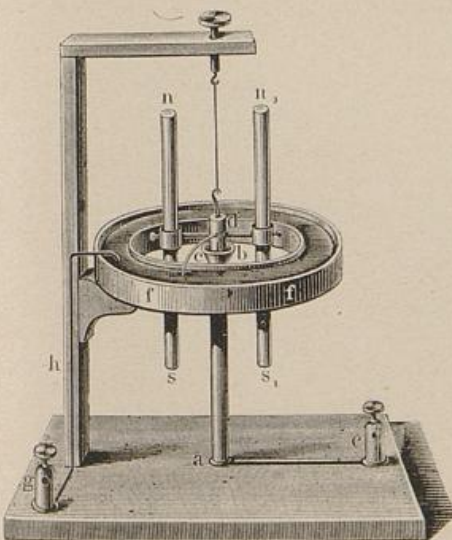
Fig. 3-5. Elektrische Rotationsapparate.
