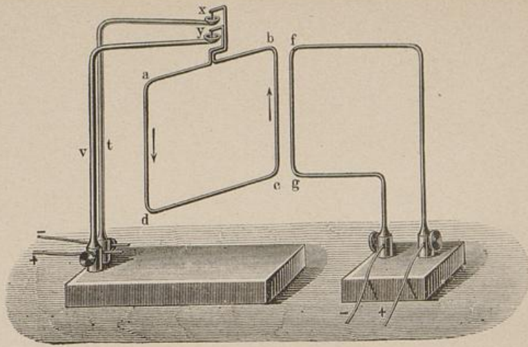
Fig. 1. Ampère'sches Gestell.
