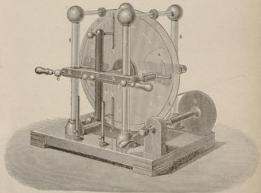
Fig. 7. Elektrische Maschine.
