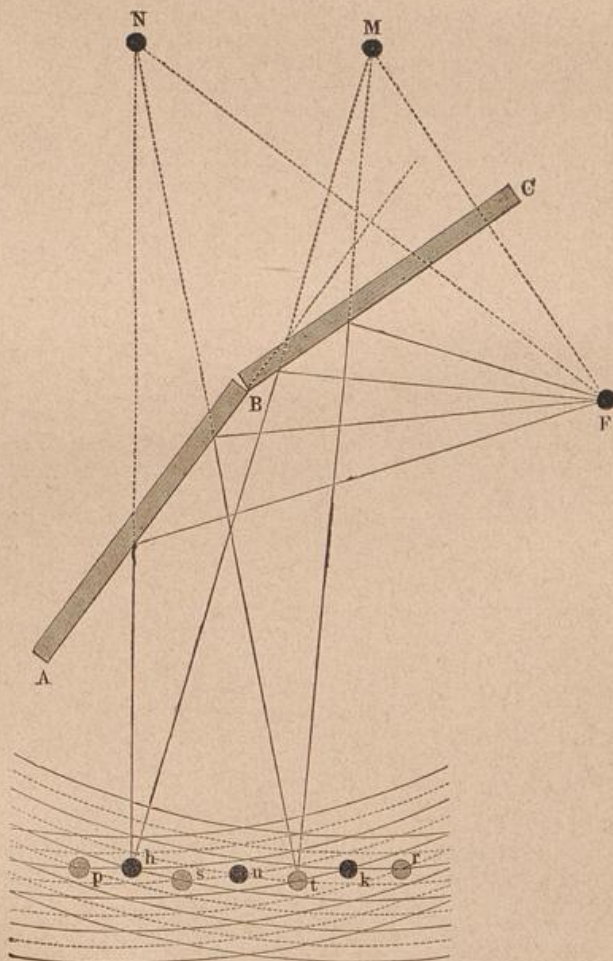
Fig. 2. Schematische Darstellung der Interferenz zweier Lichtwellensysteme.
