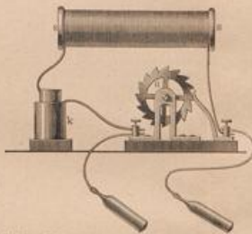
Fig. 5—6. Göttinger Apparat.
