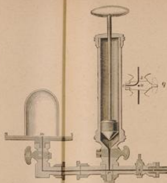
Fig. 1. Einfachwirkende Dampfkraftmaschine, Seitenansicht.
