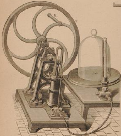
Fig. 5. Dampfschiff's doppelwirkende Dampfkraftmaschine.
