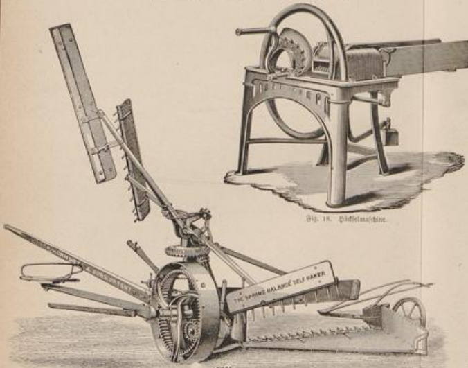
Fig. 11. Neue verbesserte füllfähige Sämaschine 'Spring Balance' von Howard.
