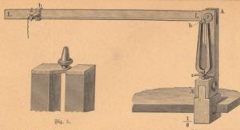
Fig. 4 Teil des Schwingenapparats. Fig. 5 die Spitze der Schwingenpfeil in größerem Maßstab.
