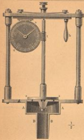
Fig. 1-3 Sirene nach Gay-Lussac de la Zener. AA die Röhre, an deren Ende; Fig. 1 Hängeschilder durch die Mitte. Fig. 2, Hängeschilder der Röhre nach der Seite aus in Fig. 2.
