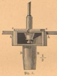
Fig. 1-3 Sirene nach Gay-Lussac de la Zener. AA die Röhre, an deren Ende; Fig. 1 Hängeschilder durch die Mitte. Fig. 2, Hängeschilder der Röhre nach der Seite aus in Fig. 2.
