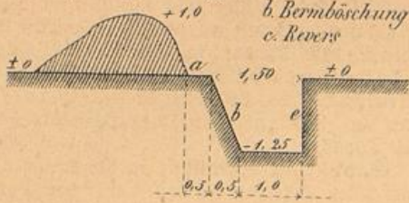
Fig 3. Profil einer Parallele mit Bankellstufen.
