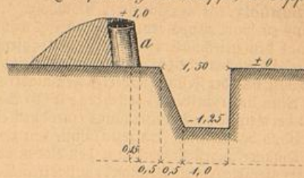
Fig 2. flüchtige Korbsappe, a. Sappenkorb
