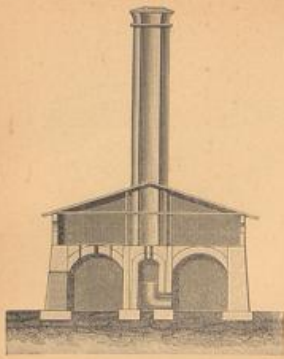
Fig. 3. Klinger Ofen, Längsschnitt.
