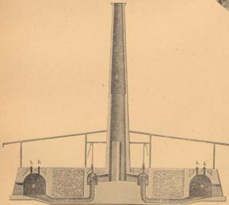
Fig. 1. Ofen, Längsschnitt.
