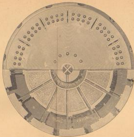
Fig. 2. Fertiger Ofen, Querschnitt.
