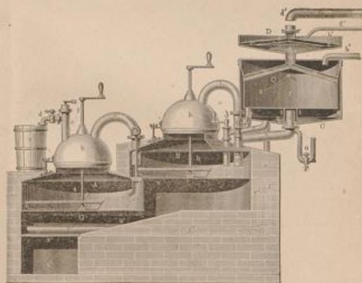
Glaskessel-Apparat zur Herstellung von Glas. A und B Heizkessel, C Heizkessel mit Heizkessel, D Heizkessel, E Heizkessel, F Heizkessel.
