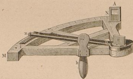
Fig. 2. Spiegelfertant einfachster Construction
