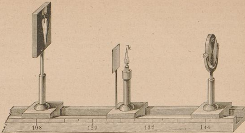
Fig. 1. Hohlspiegel, welcher das umgekehrte Bild einer Flamme k auf einen Schirm wirft.
