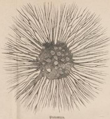
Radiolaria.
