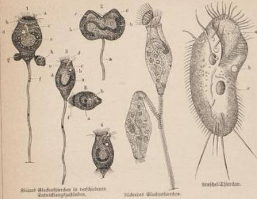
Einzelne Gladinthierien.
