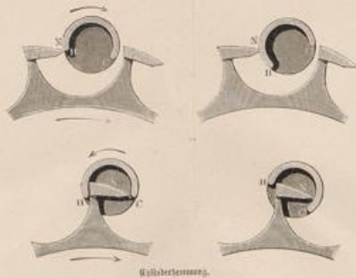
Kylinderhemmung.
