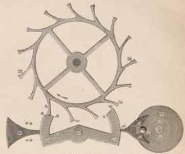
Freie Kylinderhemmung.
