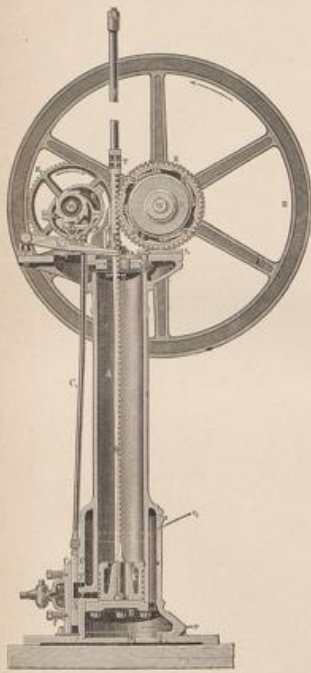
Gasmaschine.
