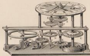
Uhr mit Spindelhemmung.
