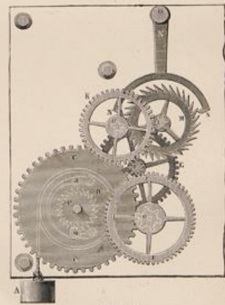
Festkette.
