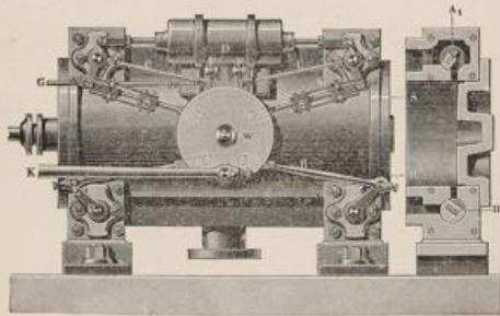
Gerät Dampfmaschine.
