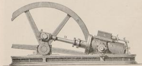
Gerät Dampfmaschine.
