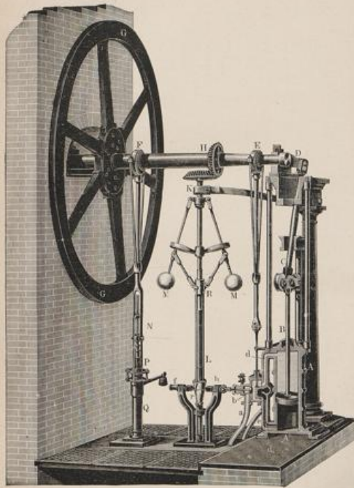
Dampfmaschine ohne Condensator.
