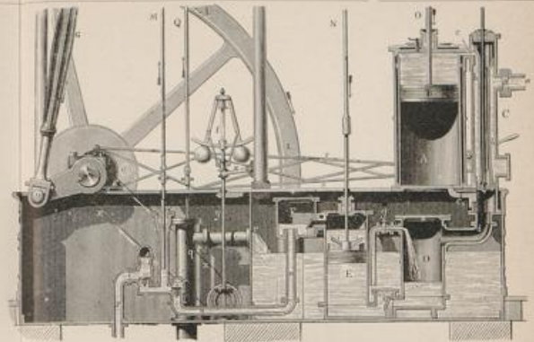
Condensierende Dampfmaschine.
