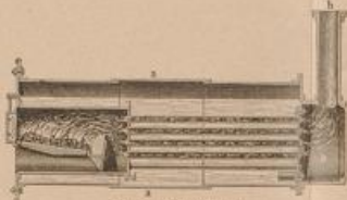
Fig. 6. Kessel-Querschnitt.
