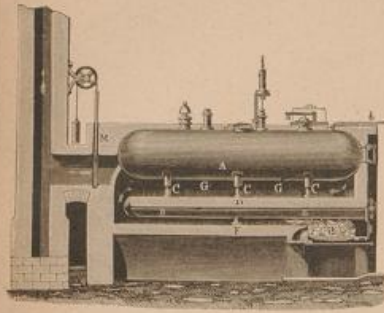
Fig. 2. Dampfessel-Querschnitt.
