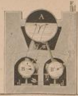
Fig. 3. Dampfessel-Crosschnitt.
