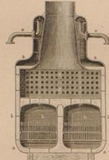
Fig. 5. Schiefen Dampfessel.
