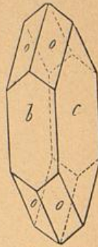
3. Combination von: Brachypinacoid (e) Macropinacoid (b) Pyramide (o). (Desmin.)
