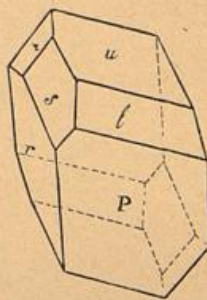
7. Combination von: Macropinacoid (r), Hemipyramid (P), 2 Viertelpyramiden (l u. u), Macropyrism s, Hemidome x. (Aeginit.)
