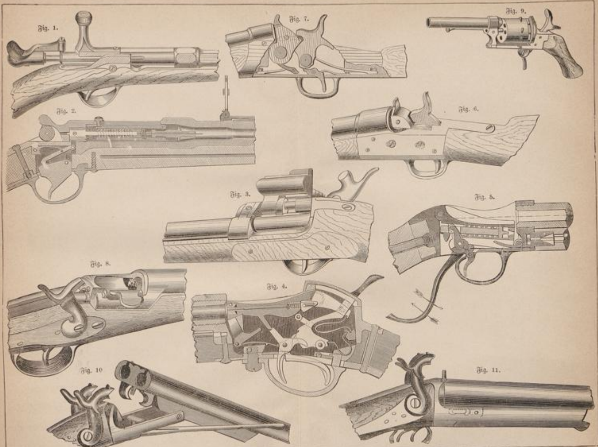
Fig. 1 und 2. Dreyfußiges Schloßsystem. 1. Geschloß und gespannt, 2. Geschloß und abgefeuert. — 3. Seiten Revolver. Zum Laden geöffnet. — 4. Büschel Revolver. Geschloß und gespannt. — 5. Englisches Patent-Revolver. Geschloß und gespannt. — 6. Revolver-Revolver. Geschloß und abgefeuert. — 7. Revolver-Revolver. Geschloß und abgefeuert (Zurückgefallen). — 8. Colverrevolver-Revolver. Geschloß und gespannt. — 9. Revolver von Ketchikan. — 10. Revolver-Revolver zum Laden geöffnet. — 11. Revolver-Revolver. Geschloß und gespannt.
