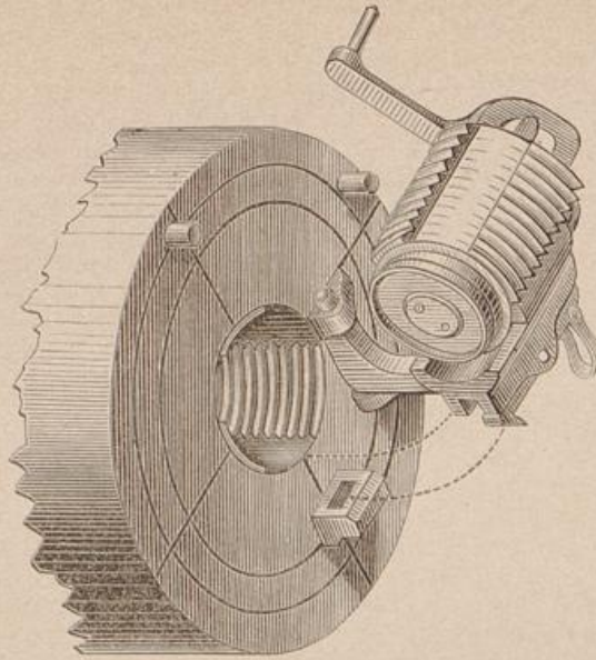
Fig. 11. Franz. Schraubenverschluß.
