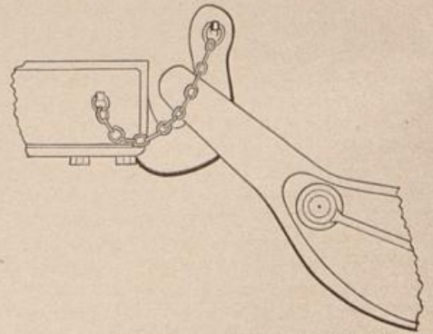
Fig. 14. Verbindung der Lafette und Prohe durch Ketten und Deise (Unabhängigkeitssystem).
