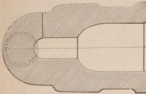
Fig. 12. Glattes Mörserrohr.
