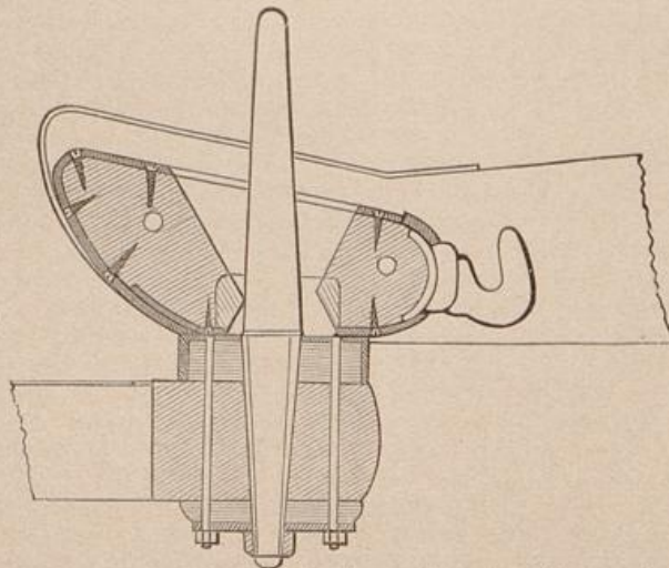
Fig. 13. Verbindung der Lafette und Prohe durch Prognagel und Proglöch (Balancier-system).
