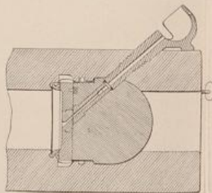
Fig. 9. Mündungsschloß (Klingenschnitt).
