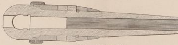
Fig. 4. Mündungsschloß (Klingenschnitt).
