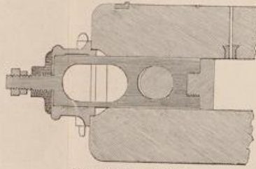
Fig. 6. b) Mündungsschloß geschlossen.
