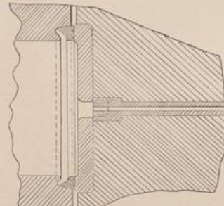
Fig. 10a. Verschlussring mit Stahlschloß.
