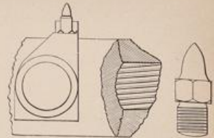
Fig. 5. Mündung auf dem rechten Schloßkopf.
