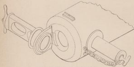
Fig. 6. Mündungsschloß. a) Mündung (geöffnet).
