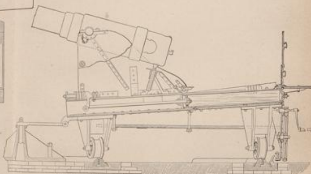
15 cm Krupp-Geschütz in der Kisten-Gefahr. Typus der deutschen Kisten-Geschütze.
