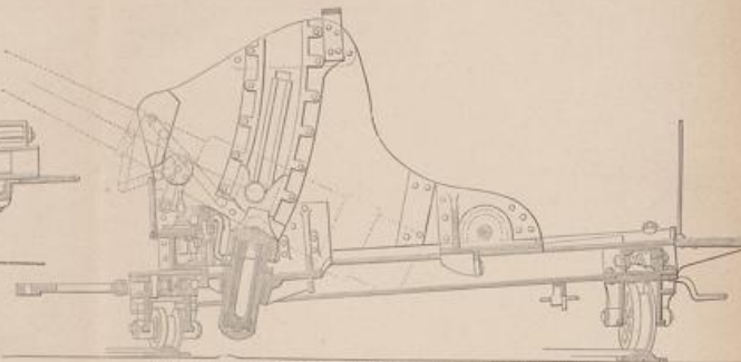
15 cm Krupp-Geschütz für 15 cm Krupp-Geschütze, zur Befestigung hinter Eisenpanzer. Nach der Construction von Krupp.
