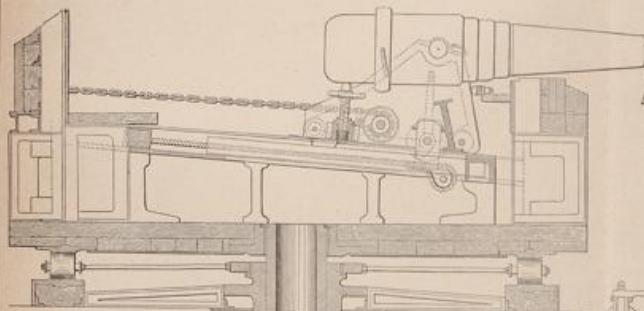
21 cm Krupp-Geschütz in der Thurm-Gefahr als Typus der Thurm-Geschütze der deutschen Marine.
