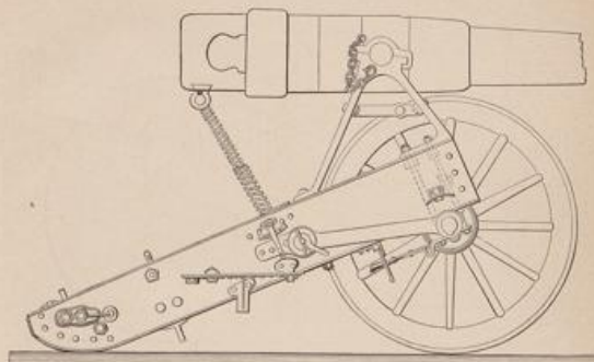
15 cm Ringkanone in der ersten Variante 1879. Typus der neuen deutschen Belagerungs-Kanonen.
