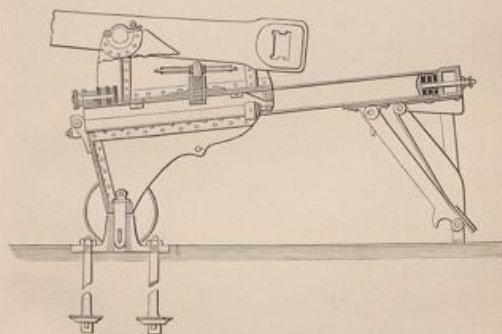
Neue deutsche Ringkanon-Kanonen-Variante vom Jahre 1879.
