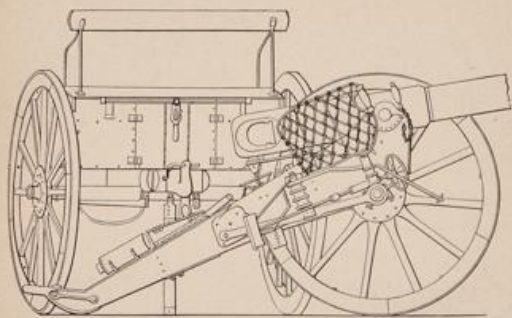
Deutsches schweres Feldgeschütz. Construction vom Jahre 1873.
