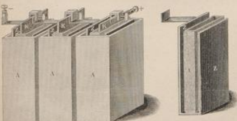
Fig. 8. Schenck'sches Galvanometer.
