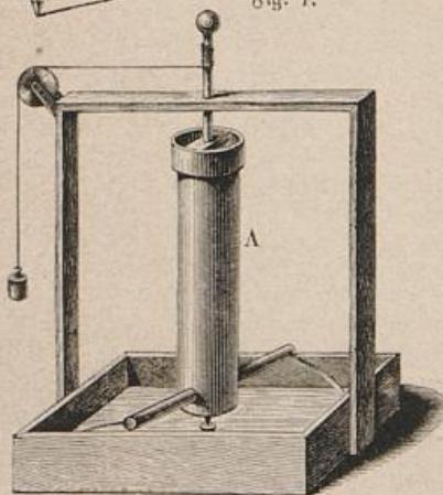
Fig. 4. Segner'sches Wasserrad.
