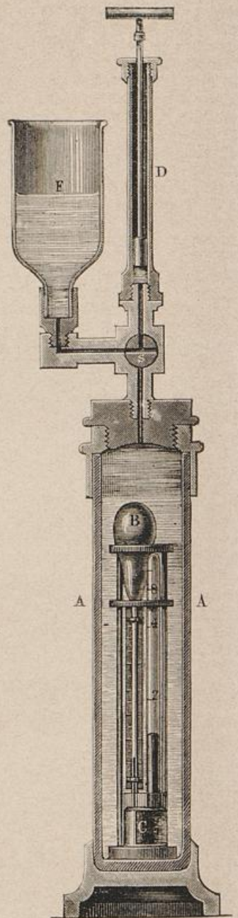
Fig. 3. Piezometer.
