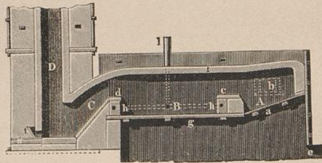
Puddlingsflammofofen, Längsfchnitt.
