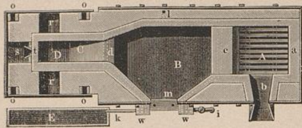
Puddlingsflammofofen, Horizontalfchnitt.
