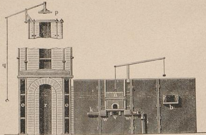
Puddlingsflammofofen, Anficht.
