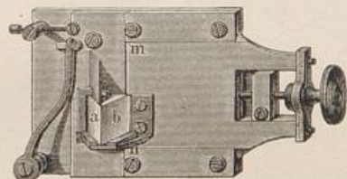
Fig. 2. Vergleichsprisma zum Spectralapparat.
