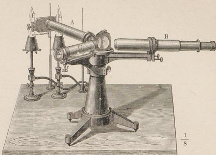
Fig. 1. Spectralapparat.
