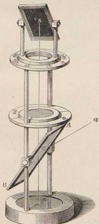
Fig. 4. Nörrenberg'scher Polarisationsapparat.
