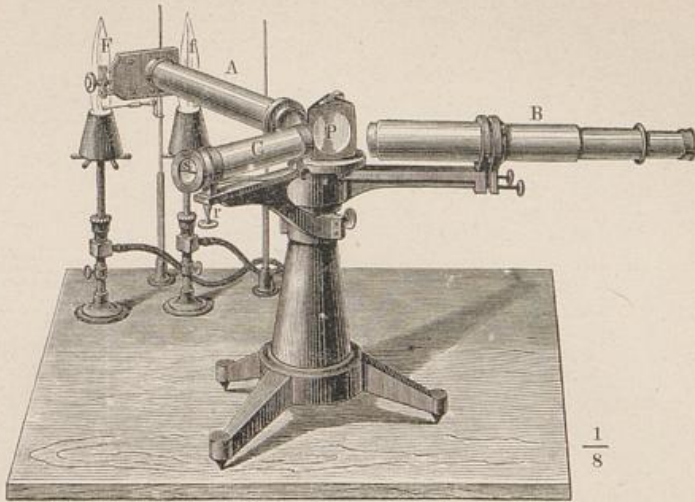
Fig. 1. Spectralapparat.
