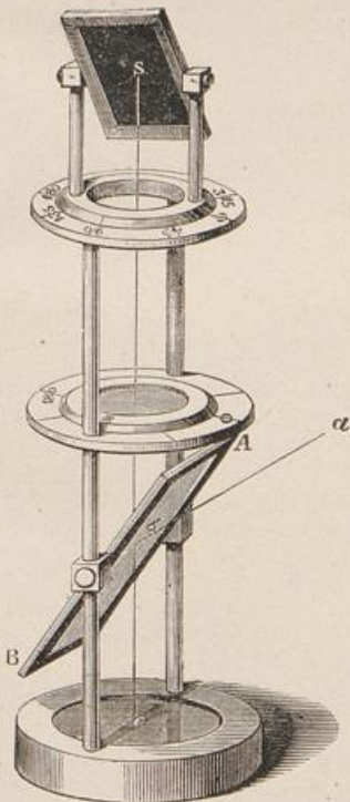
Fig. 4. Nörrenberg'scher Polarisationsapparat.
