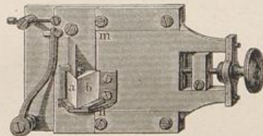
Fig. 2. Vergleichsprisma zum Spectralapparat.
