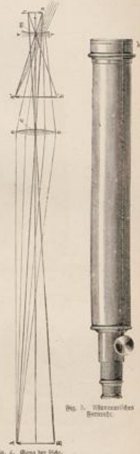
Fig. 6. Gang der Lichtstrahlen im Copier des hessischen Fernrohrs.
