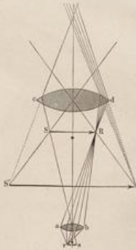
Fig. 11. Gang der Lichtstrahlen im Mikroskop.
