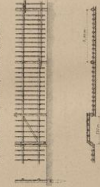
Fig. 73b. Leichter Lattenzaun, geschnitten u. gestügelt.
