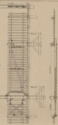
Fig. 73d. Drehbarrere
