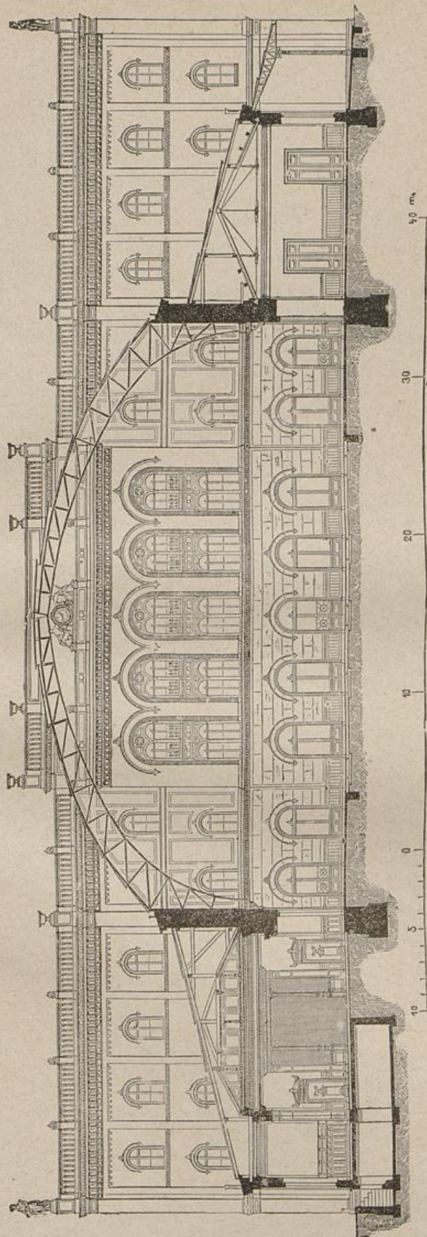
Fig. 71. Beigt als Beispiel, wo sämtliche Perrons und Geleise überdeckt sind, die Halle der Ostbahn zu Berlin.
