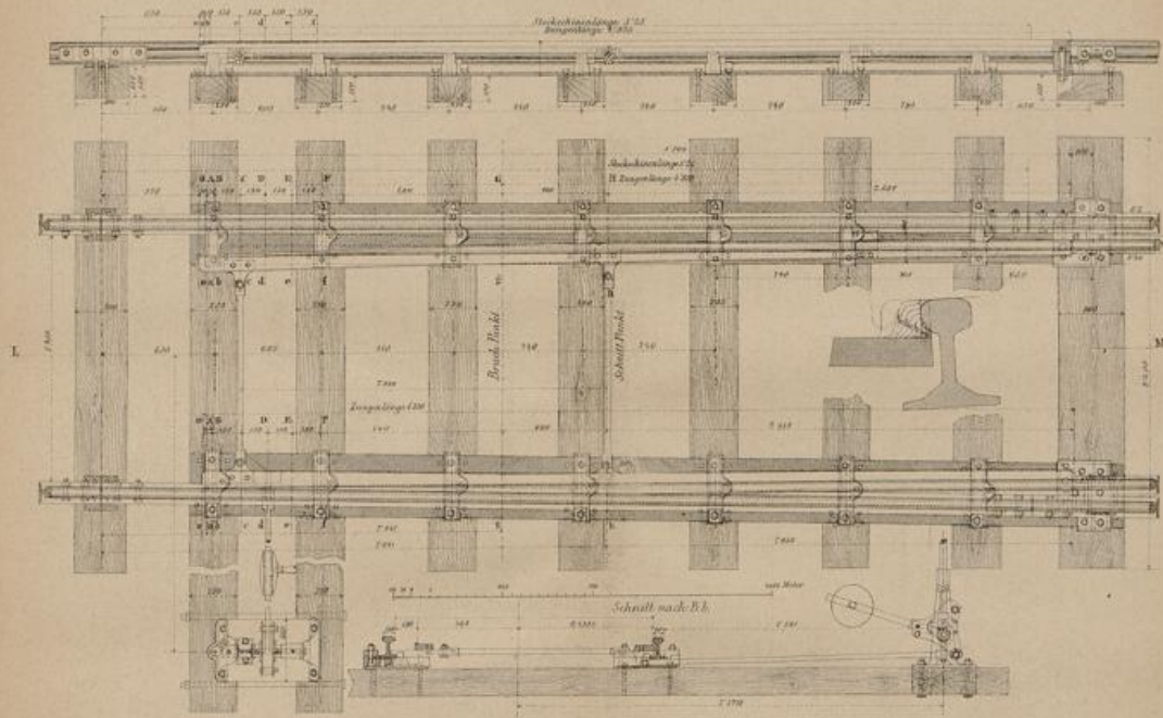
Fig. 51. Einfache Weiche.
