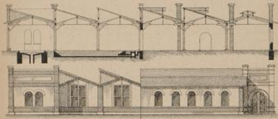
Fig. 67. Werkstätte.
