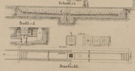
Fig. 72. Putzgrube.
