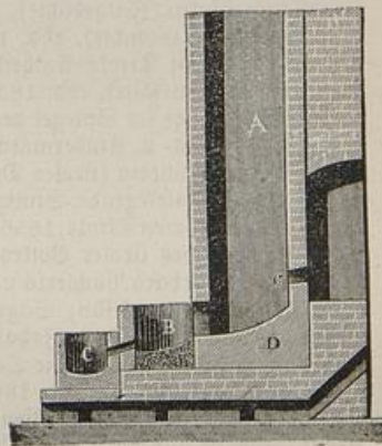
Fig. 7. Zinn-Schachtofen. Querschnitt.
