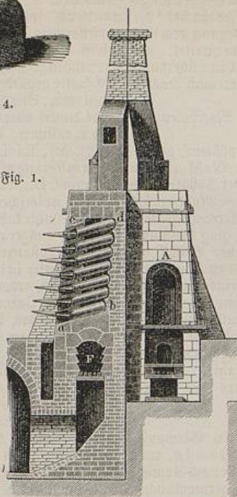
Belgischer Zinkofen.
