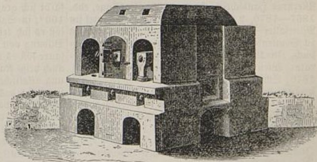
Fig. 3. Schlesischer Zinkofen. Ansicht.
