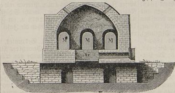
Fig. 4. Schlesischer Zinkofen. Querschnitt.
