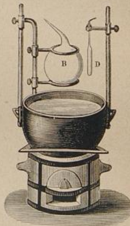
Fig. 2. Apparat von Dumas zur Bestimmung der Dampfdichte.
