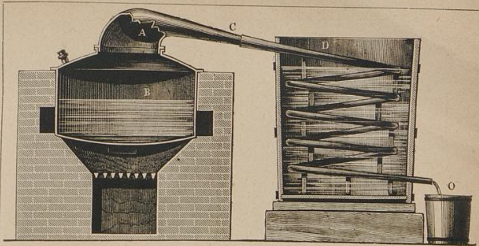
Fig. 1. Destillationsapparat.
