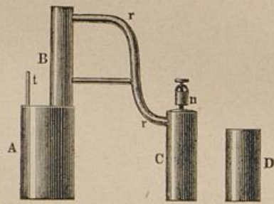
Fig. 3. Carré's Eismaschine für Ammoniak.
