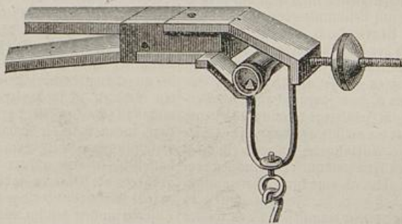
Fig. 2. Aufhängung der Wagechalen von Fig. 1.
